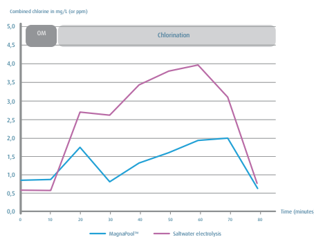
Křivka poklesu vázaného chlóru oproti slané vodě
