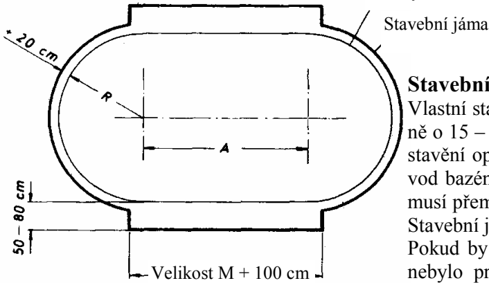
Půdorys bazénu
