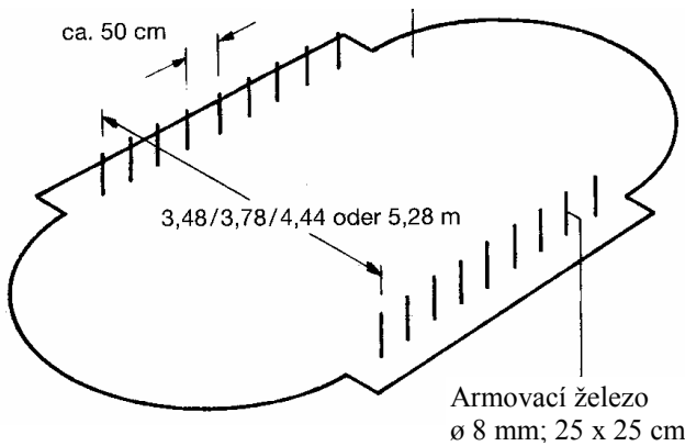
Betonová základová deska
